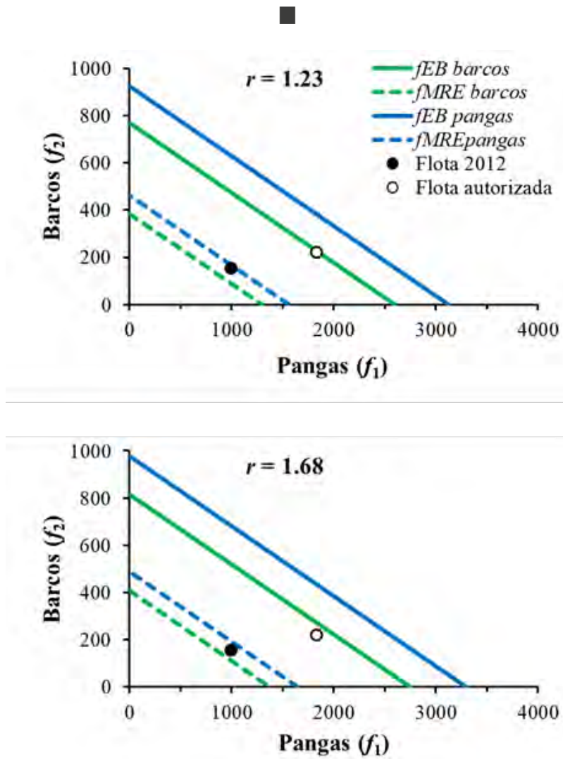
Gráfica 3. Isoclinas bioeconómicas del modelo de dos flotas compitiendo por un stock: a) r = 1.23 y b) r = 1.68 .
